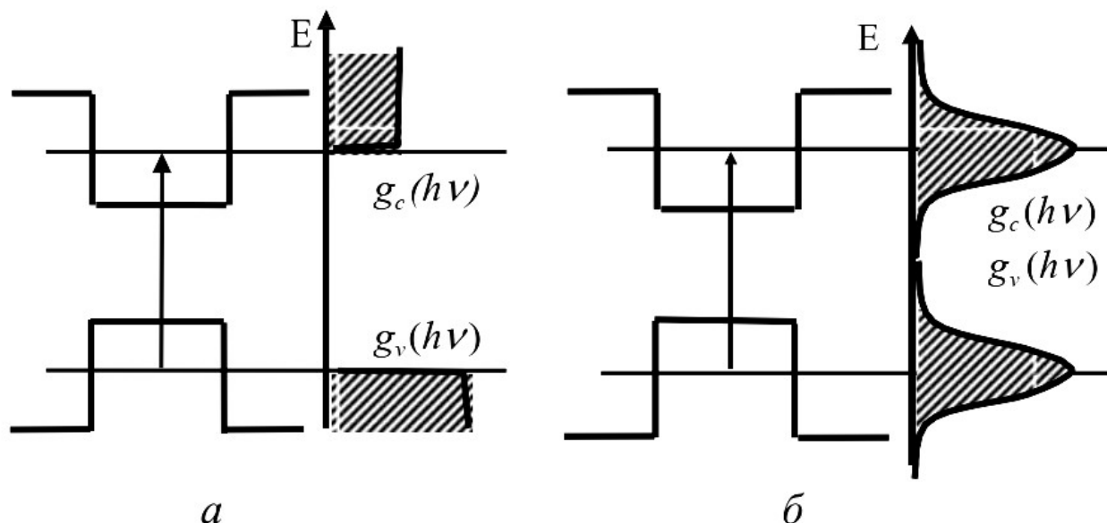
1-rasm. GeSi/Si kvant-o‘ra tuzilmalarida elektron holatlar zichligining energiya taqsimoti [8]: a – kvant o‘ra, b – kvant nuqta.
