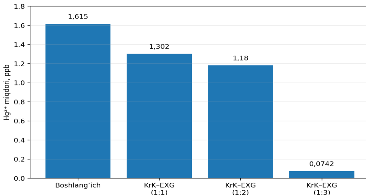
3-rasm. KrK-EXG tarkibiga bog' liq holda oqova suvdagi qoldiq Hg 2+ miqdorining o' zgarishi
