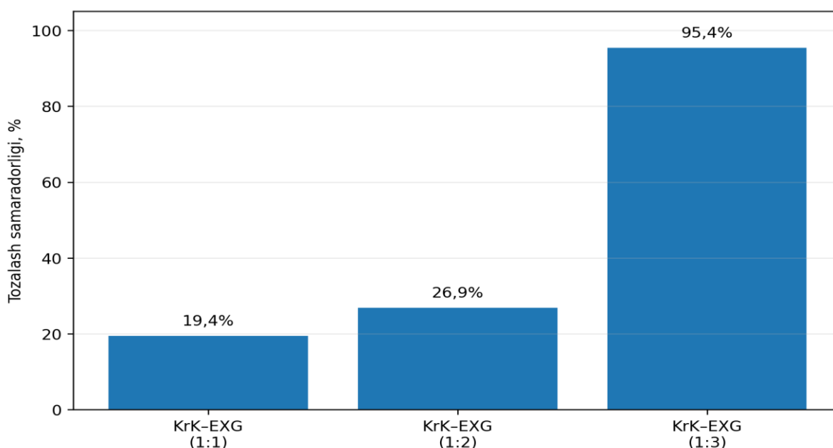
4-rasm. KrK-EXG sorbentlari bilan Hg 2+ ionlarini chiqarib tashlash samaradorligi
