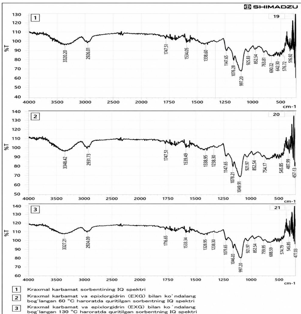
2-rasm. - Kraxmal karbamat va uning epixlorgidrin (EXG) bilan ko'ndalang bog'langan hosilalarining IQ-spektrlaridagi strukturaviy o'zgarishlar: 1 — kraxmal karbamat; 2 — epixlorgidrin bilan ko'ndalang bog'langan va 60 °C da quritilgan KrK-EXG sorbenti; 3 — epixlorgidrin bilan ko'ndalang bog'langan va 130 °C da termik ishlov berilgan KrK-EXG sorbenti.
