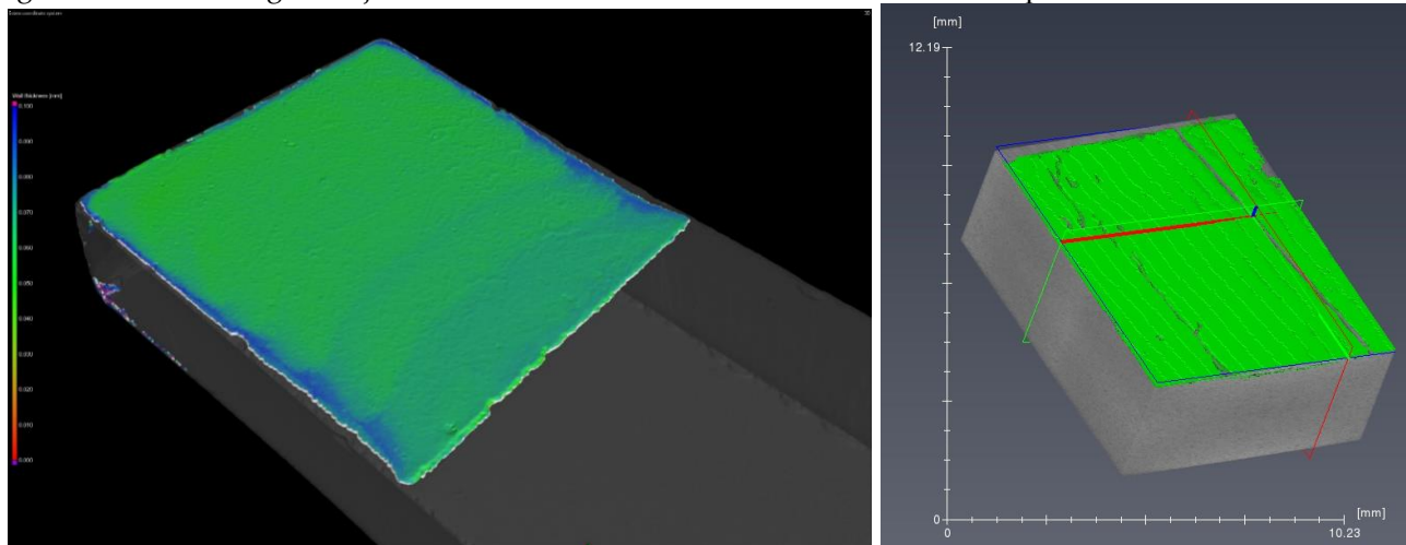
1-rasm. Ikki qatlamli (chapda) va bir qatlamli (o' ngda) \text{TiO}_2 fotoanodlarning dastlabki rekonstruksiyalari [1].
