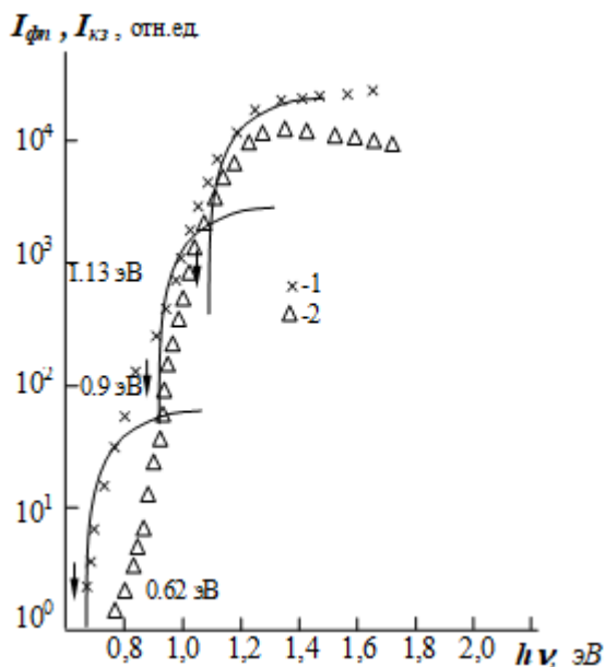
Рис.2. Спектры тока фотопроводимости (кривая 1) и тока короткого замыкания (2) пленок CdTe:Ag , полученных при скорости конденсации 0,3 \text{ нм/с} . T = 300^{\circ} \text{ K} .
