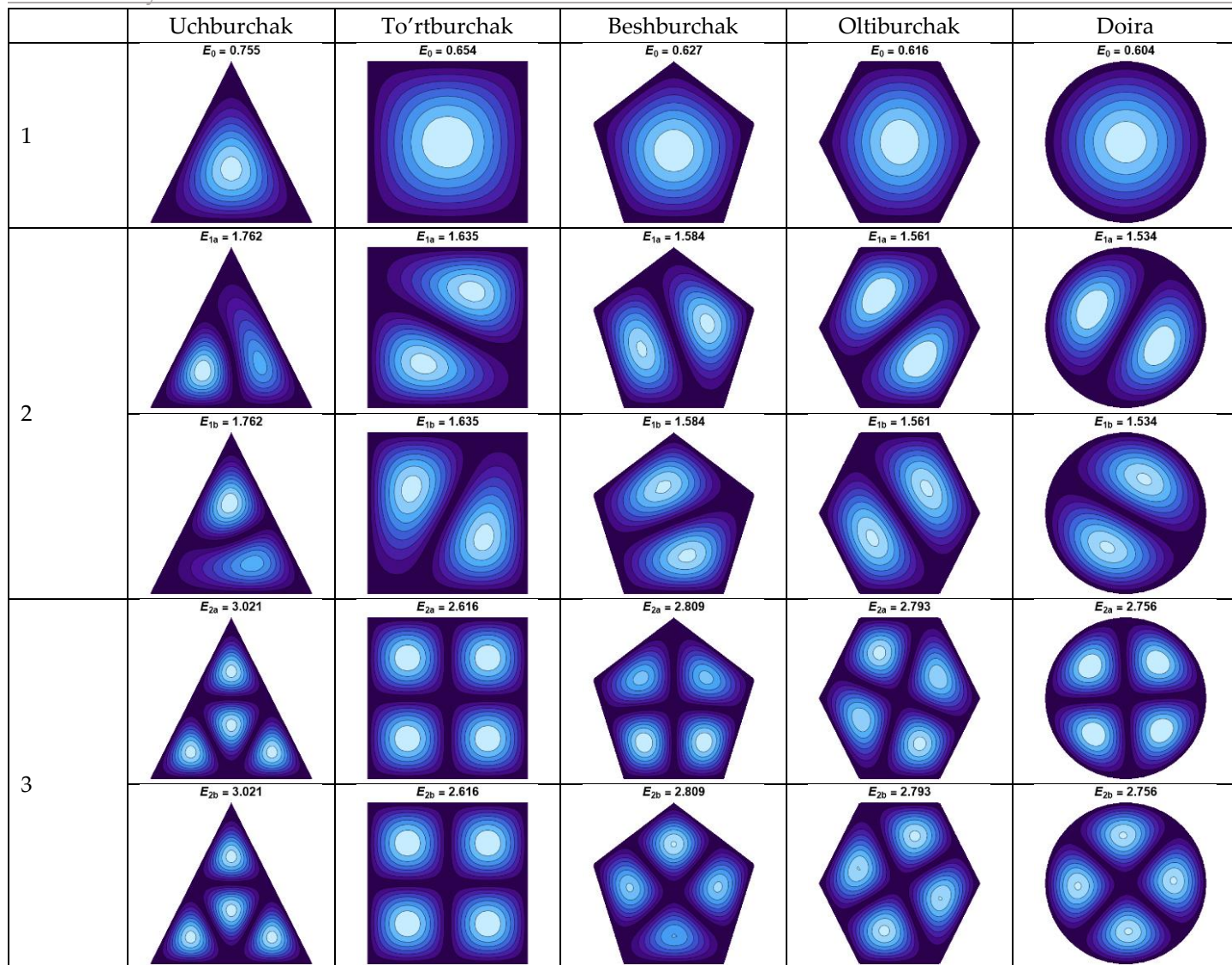
5-rasm. Asosi muntazam qabariq uchburchakli, to'rtburchakli, beshburchakli, oltiburchakli va doiraviy shaklda bo'lgan nanoiplarda to'liqin funksiyalarni 2D tasviri.
