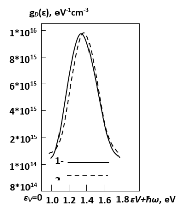
Рис. 4. Рассчитанные распределения плотности электронных состояний D^+ дефекта 1 - по формуле (19), 2 - по формуле (20).
