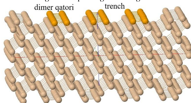
1- rasm. Kremniy taglikdagi dimer va trench qatorlari
