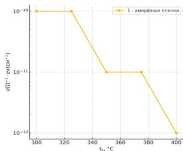
Рисунок 3: Зависимость проводимости аморфных пленок ZnO:B от температуры подложки
