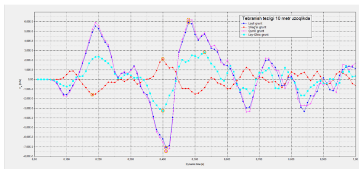
3-rasm. Turli xil gruntlarda temir yo'l chetidan 10 m masofadagi tugunlarda hosil bo'ladigan X o'qidagi tebranish tezligining vaqtga bog'liq grafifi
