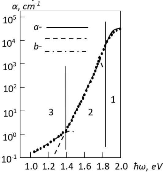
Рис. 2. Экспериментальный спектр \alpha -Si:H. Где участки 1 – межзонного, 2 – экспоненциального, 3 – дефектного поглощения. Рассчитанные спектры оптического поглощения \alpha -Si:H a – межзонное поглощения, b – экспоненциального поглощения, c – дефектного поглощения.
