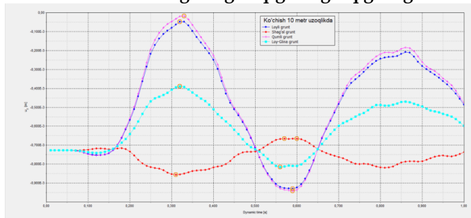
4-rasm. Turli xil gruntlarda temir yo'l chetidan 10 m masofadagi tugunlarda hosil bo'ladigan Z o'qidagi kochishlarni vaqtga bog'liq grafifi
