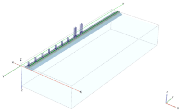
b) temir yo'lining joylashuvi va tanlangan cheklangan hududda yukning harakatlanishi
