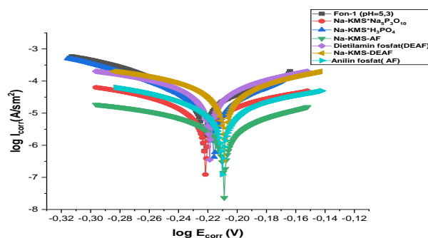
3-rasm. Qutblanish egrilari usuli yordamida olingan natijalar fon eritmasi pH=5,3 (5%Na 2 SO 4 +3%H 2 SO 4 ) li muhitda 30 mg/l miqdorda turli ingibitorlarni kiritilgandagi natijalari Fon (1); Na-KMS·Na 5 P 3 O 10 (2); Na-KMS·H 3 PO 4 (3); (Na-KMS+AF) (4); DEAF (5); (Na-KMS+DEAF) (6); AF(7).
