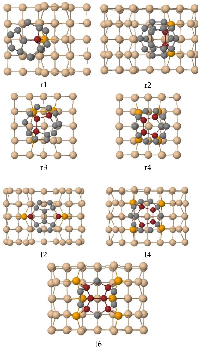
2- rasm. C_{20} fulleren molekulasining kremniy Si(001) sirtida dimer qatorlari va trenchda adsorbsiyalanish holatlarining yuqoridan ko'rinishi
