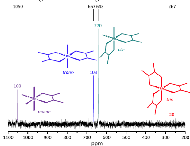
3-rasm. H_2O_2 bilan 2 soat qaynatilgandan keyin Rh(OH)_3 ni H_2O da eritib olingan eritmaning ^{103}Rh NMR spektri
