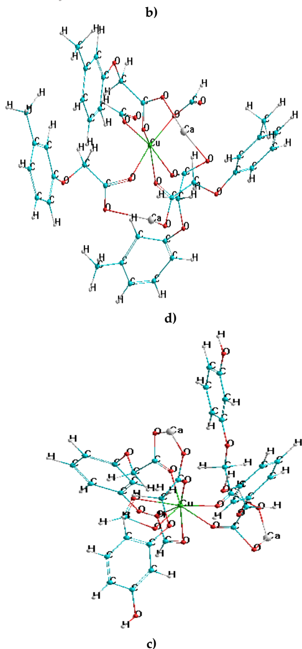
4-rasm. Kompleks birikmaning 1:1 nisbatdagi koordinatsion soni 4 (a) va 6 (b) hamda 1:2 nisbatdagi koordinatsion soni 6 (c) va 8 (d) ga teng bo'lgan kvant-kimyoviy modellashtirishdan olingan fazoviy tuzilishlari
