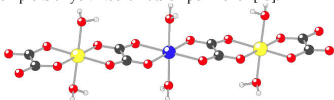
2-rasm. Tashqi sferadagi suv molekularini ko'rsatmasdan [M(H_2O)_2(m-Ox)Rh(H_2O)_2Ox]_2 \cdot 6H_2O kompleksining tuzilishi.
