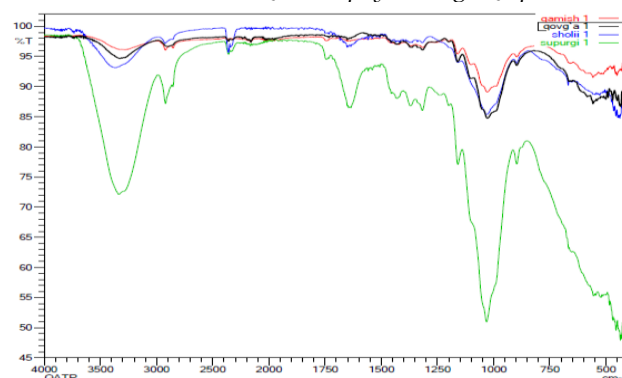
3-rasm Bir yillik o'simliklar poyasidan ajratib olingan selluloza na'munalarining solishtirilgan IQ spektrlari
