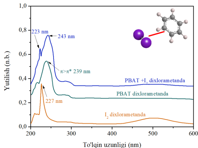
2-rasm. Dixlorometanda eritilgan I 2 , PBAT hamda PBAT+ I 2 ning ultrabinafsha va ko'zga ko'rinuvchi spektral sohalardagi yutilish spektrlari. Yuqori o'ng burchakda benzol halqasi va I 2 ning o'zaro ta'sirlashish sxemasi ko'rsatilgan (binafsha shar- I, kulrang shar-uglerod, oq rang-vodorod).
