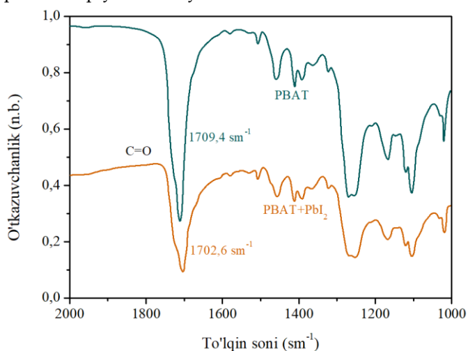
1-rasm. PBAT va PBAT-PbI 2 ning IQ-Fure spektrlari
