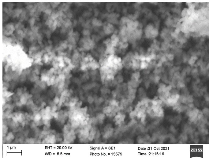
2-rasm. TiO_2 kolloid zarralari uchun SEM da olingan relieflil tasviri masshtab 1sm:1mkm
