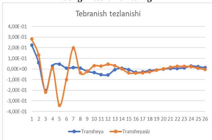
6-rasm. Temir yo'l markazidan 20 metrdan 80 metrgacha bo'lgan masofada hosil bo'lgan tebranish tezlanishi
