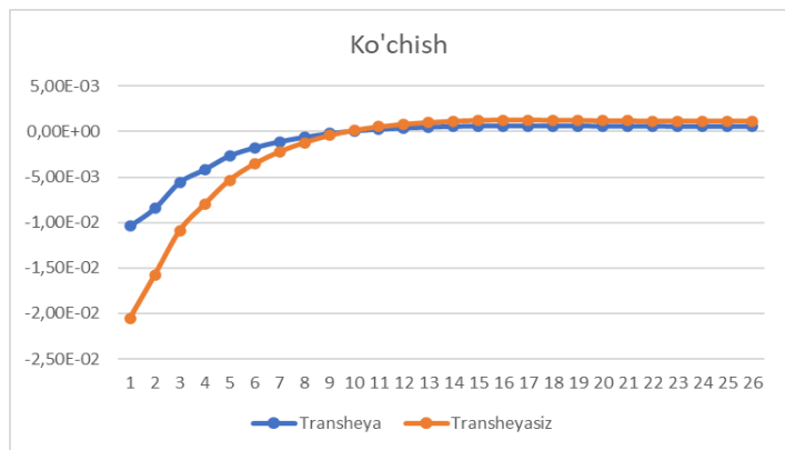
4-rasm. Temir yo'l markazidan 20 metrdan 80 metrgacha bo'lgan masofada hosil bo'lgan ko'chishlar
