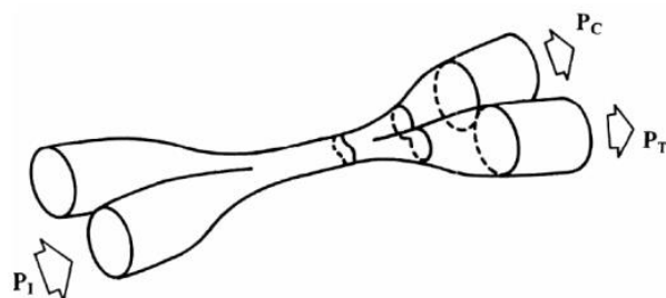
Рис. 6 Схема сплавного биконического ответвителя.
