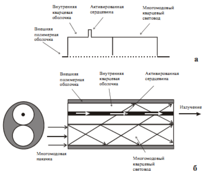
Рис.4.Профиль GTWave (генератор двухканальной волновод) волокно: (а) – модельный профиль преломления, (б) - иллюстрация перехода многомодовой накачки в активный световод и преобразования в одномодовое излучение волоконного лазера.
