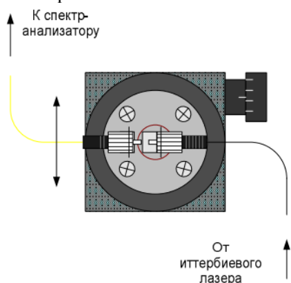
Рис. 8 Схема расположения торцов оптических кабелей лазера и приемной части на поворотном столике.
