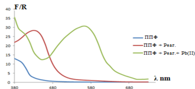
3-рис. Функция (Кубелки-Мунки) зависимости от коэффициента отражения комплекса, образованного волокном ППФ, волокном и солью АНФБ, иммобилизованным волокном и ионом Pb(II)
