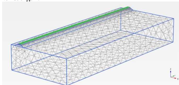
2-rasm. Tanlangan modelning cheklangan elementlarga bo'lingan holati.
