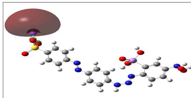
5-рис. Нижняя незанятая молекулярная орбиталь, LUMO реагента АНФБ
