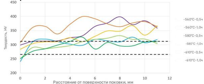
Рис. 5. Изменения твердости HV в поперечном сечении в выбранной плоскости измерения для изотермически отожженного образца
