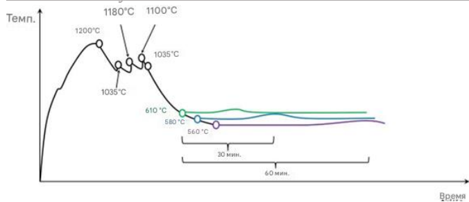
Рис. 4. Зависимость режима температуры и времени во время термомеханической обработки
