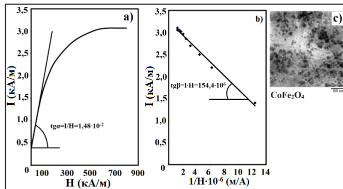
4-rasm. NiFe 2 O 4 magnit suyuqlik uchun a) I=I(H); b) I=I(1/H); c) TEM da olingan fotosurati.
