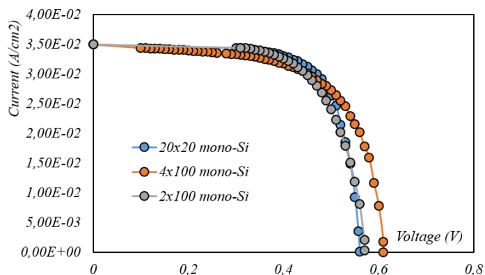
Рис. 7. Кривые ВАХ кремниевого солнечного элемента с различными геометрическими размерами 2×100 mm 2 , 4×100 mm 2 и 20×20 mm 2 , измеренные на автоматизированной установке «Sinton-Instrument Suns-V oc »
