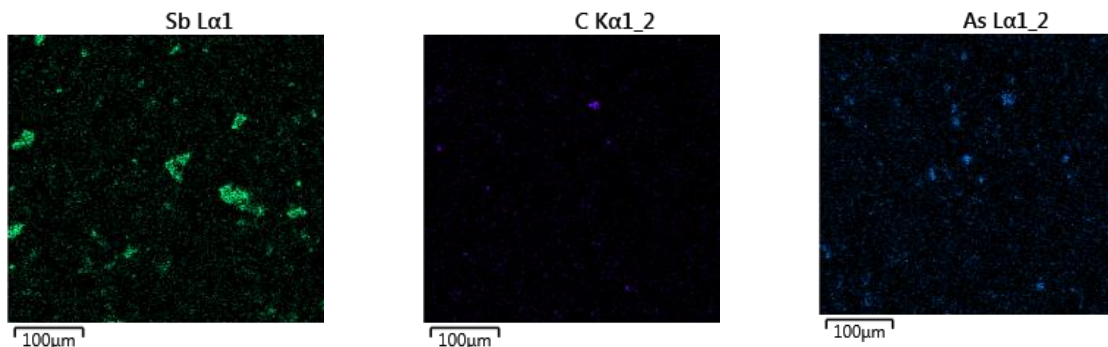
Рис. 9. Изображение №1 поверхности образца №793 полученное на электронном микроскопе с увеличением в 500 раз для получения карты по элементному составу образца
