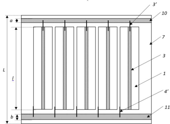
Рис. 2. Вид с веру горизонтального разреза полупроводникового фотоэлектрического гибкого модуля
