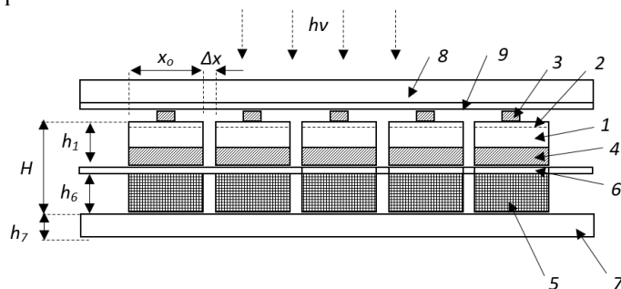
Рис. 1. Поперечный вид в вертикальном разрезе полупроводникового фотоэлектрического гибкого модуля
