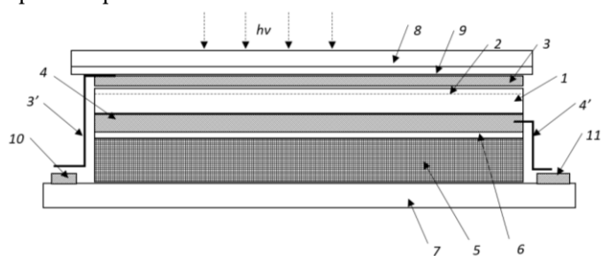
Рис. 3. Продольный вид в вертикальном разрезе полупроводникового фотоэлектрического гибкого модуля
