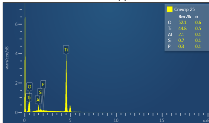
3-rasm. TiO_2 kolloid zarralari uchun SEM da olingan spektral tasviri
