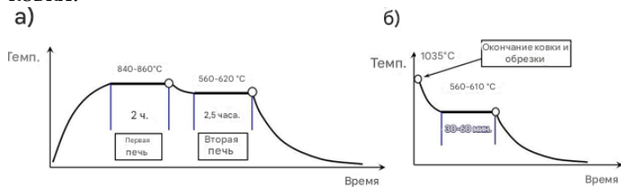
Рис. 2 а) метод термообработки со стандартным изотермическим отжигом; б) метод термообработки изотермическим отжигом непосредственно послековки
