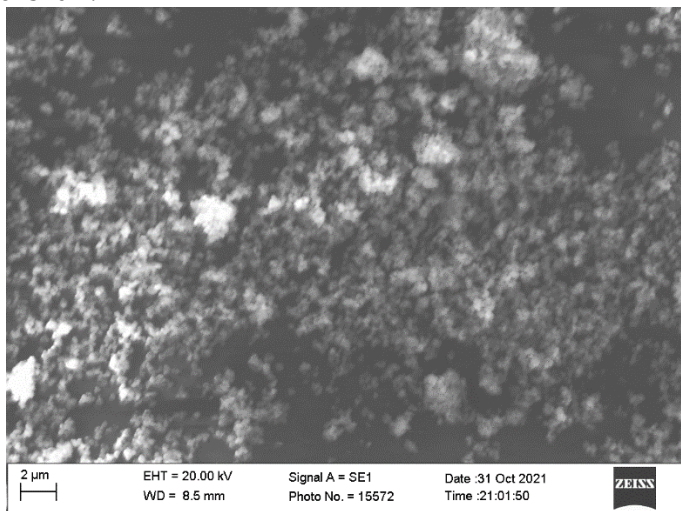
1-rasm. TiO_2 kolloid zarralari uchun SEM da olingan relieflil tasviri masshtab 1sm:2mkm
