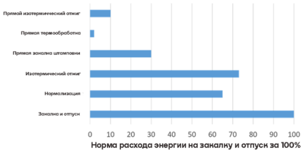
Рис.1. Зависимость энергопотребления от видов термообработки
