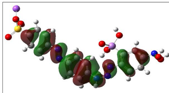
4-рис. Высшая занятая молекулярная орбиталь, НОМО реагента АНФБ
