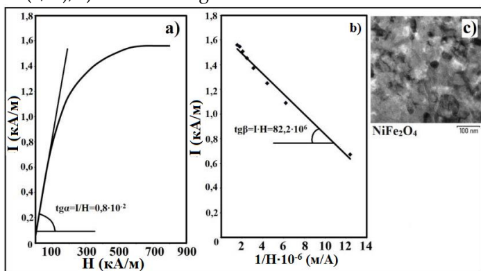
3-rasm. SoFe 2 O 4 magnit suyuqlik uchun a) I=I(H); b) I=I(1/H); c) TEM da olingan fotosurati.
