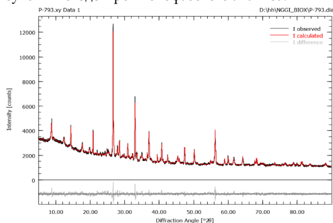
Рис. 7. Рентгенограмма образца флотоконцентрата (рН-8,2)
