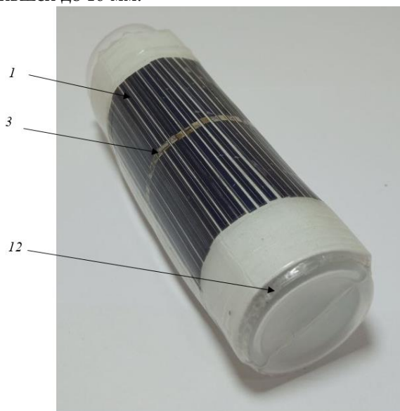
Рис. 6. Фотография опытного кремниевого фотоэлектрического гибкого модуля (без контактных шин), установленного на внешнюю поверхность цилиндрического предмета
