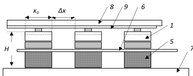
Рис. 4. Поперечный вид в вертикальном разрезе полупроводникового фотоэлектрического гибкого модуля, предусмотренного для внешней выпуклой поверхности предмета
