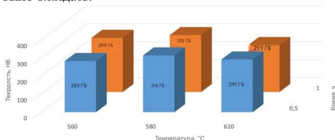
Рис. 6. Результаты испытаний по методу Бринелля средней твердости изделий из модифицированной хромомолибденовой стали для различных времен изотермического отжига и температур
